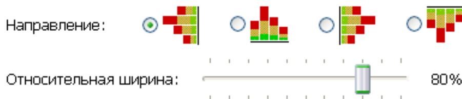
Рис.2.7. Направление столбцов
