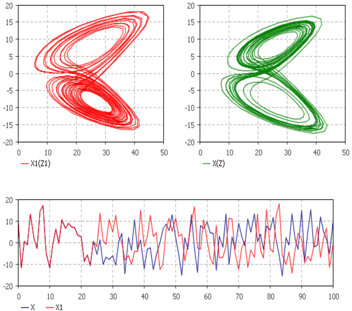
Рис.1.4. Сравнение работы двух моделей
