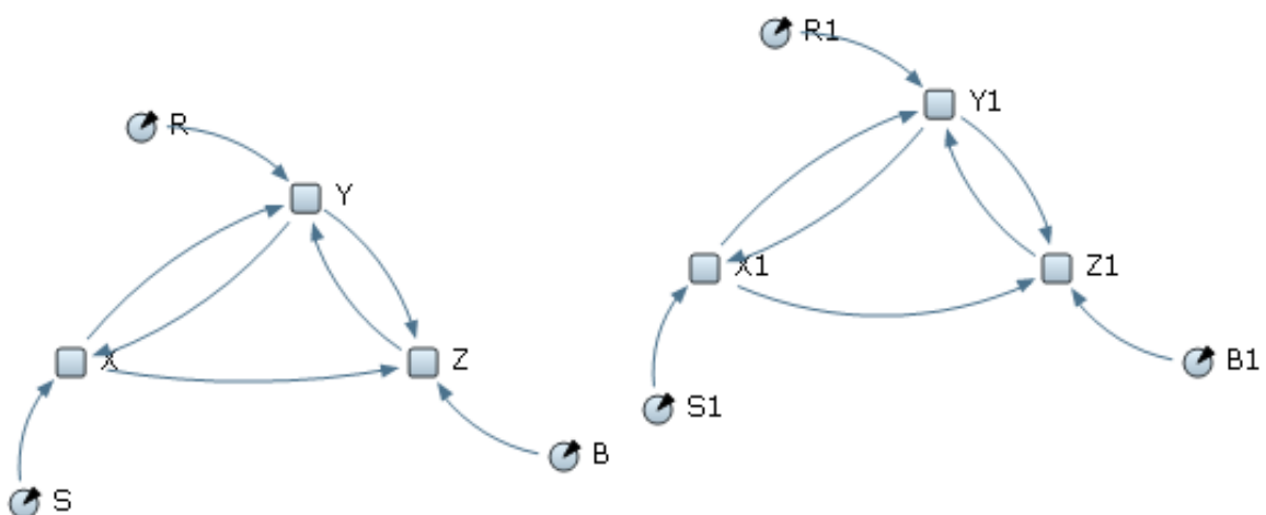
Рис.1.3. Две модели Лоренца
