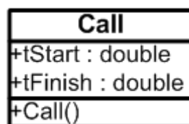
Рис.3.7. Класс Call
