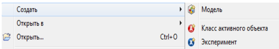
Рис. 3.9. Контекстное меню
