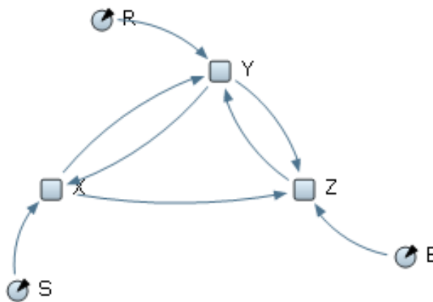
Рис.1.1. Модель Лоренца
